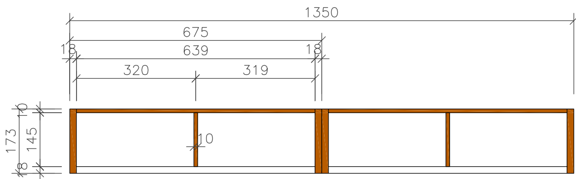
PŮDORYS
