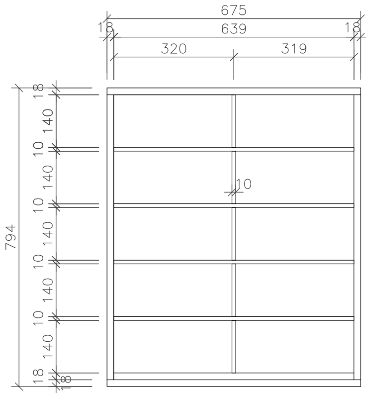
NÁRYS
