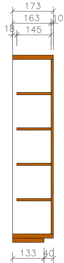
ŘEZ
